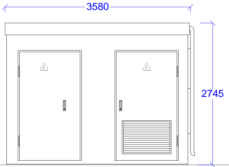
Elewacja przednia
