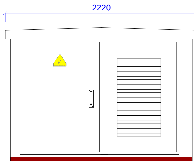
Elewacja boczna prawa
