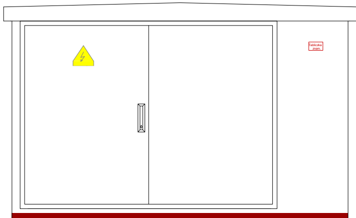
Elewacja przednia
